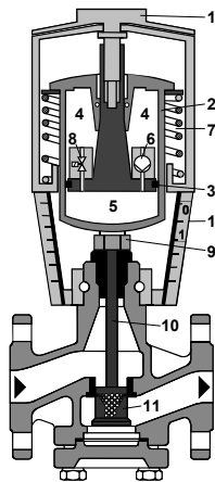
Клапан открыт
