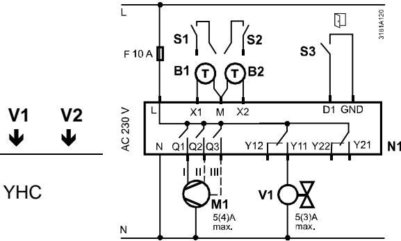
1- or 3-speed fan
