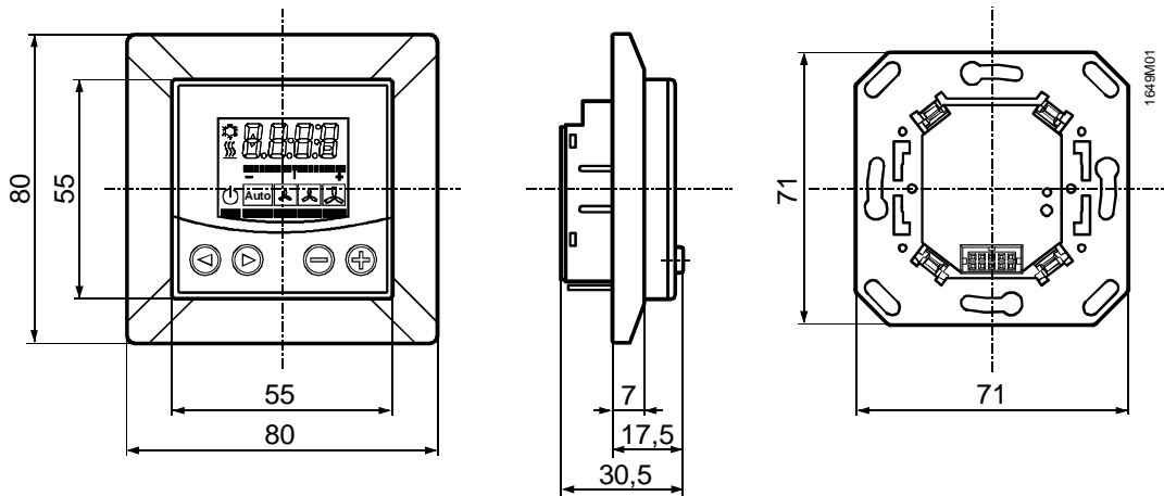
QAX84.1/PPS2 (комнатный модуль)
